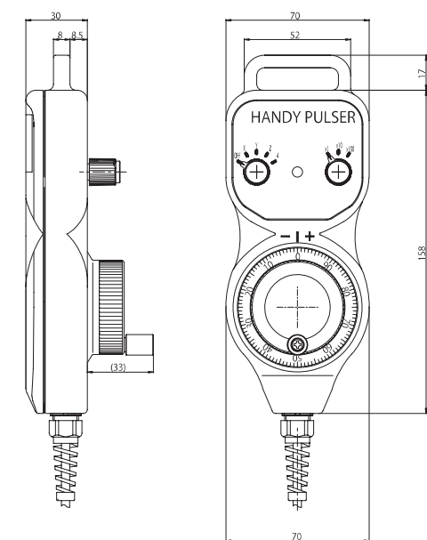
【HP-M外形図】
