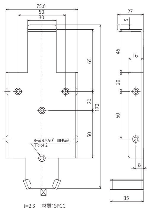
【ホルダー外形図】(別売)
